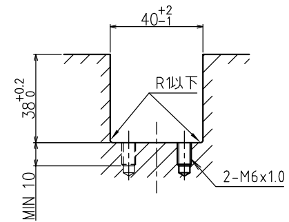
取付溝寸法図
