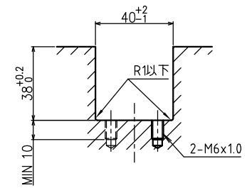
取付溝寸法図
