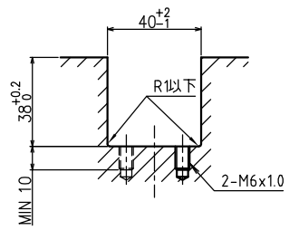
取付溝寸法図
