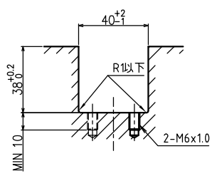
取付溝寸法図
