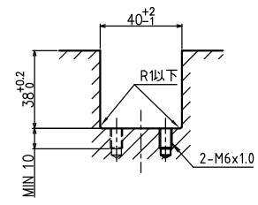
取付溝寸法図
