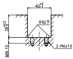
取付溝寸法図
