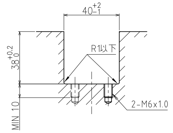
取付溝寸法図
