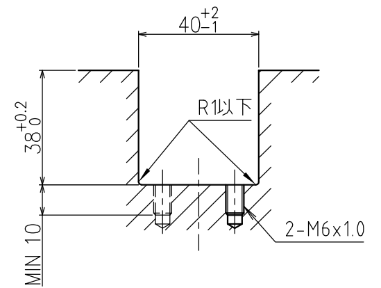
取付溝寸法図
