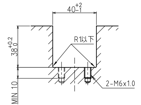
取付溝寸法図
