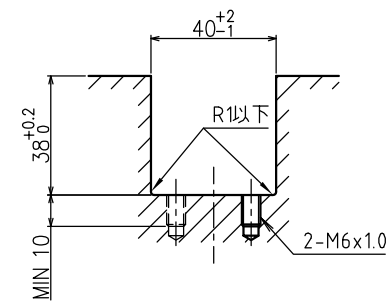
取付溝寸法図
