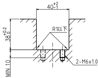
取付溝寸法図
