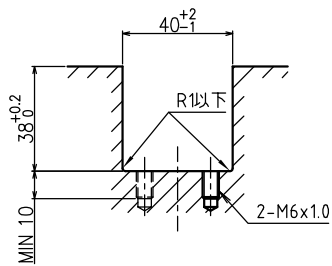
取付溝寸法図
