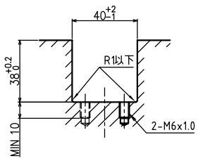
取付溝寸法図
