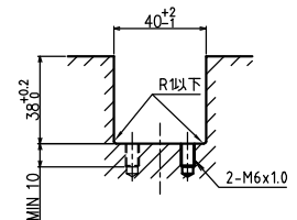
取付溝寸法図
